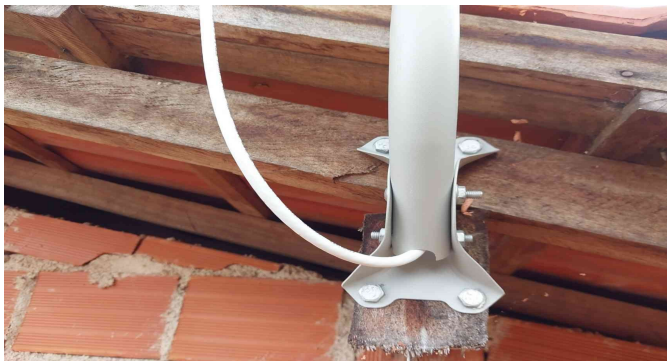
Foto – Fixação da Base da Antena
